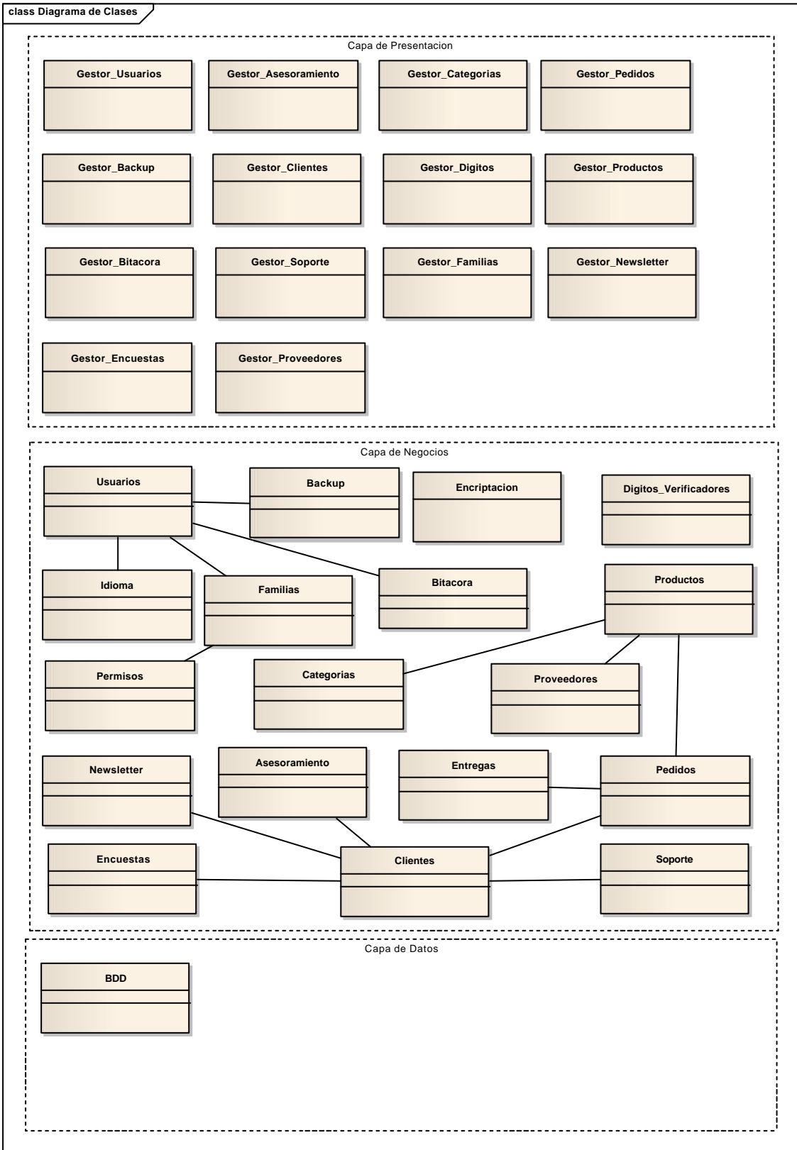
class Diagrama de Clases
