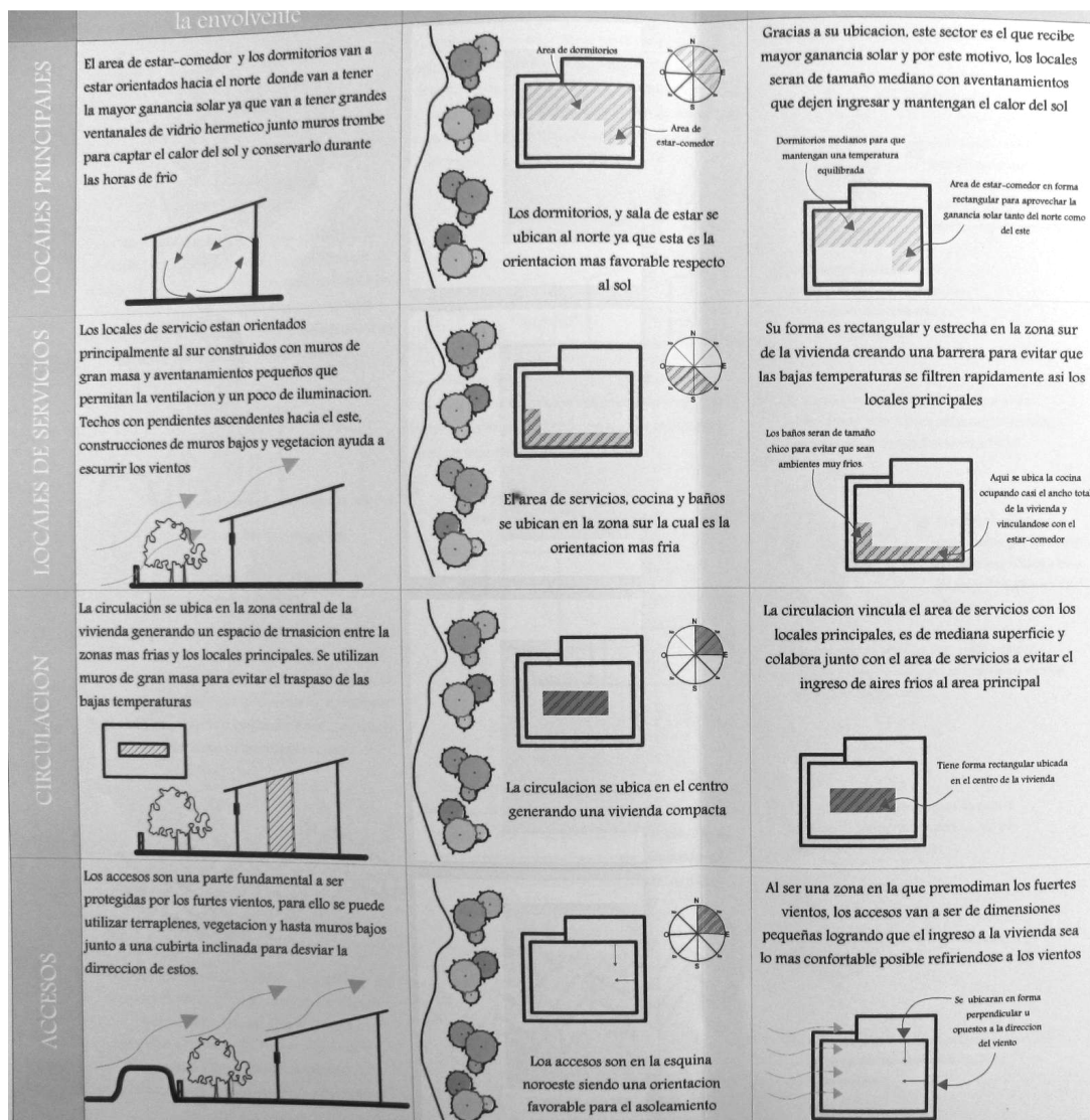
Fig. 2: Pautas de Diseño Bioclimático para la escala edilicia
