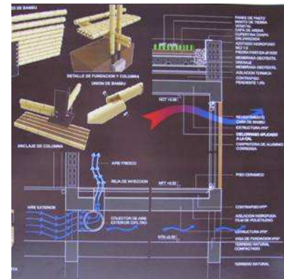
Figs. 7 y 8: Envolvente resuelta con tecnología de caña adaptada a diferentes orientaciones, generando fusión interior- exterior según la necesidad.
